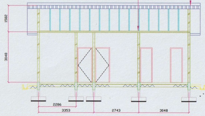
KERATAN Q - Q
