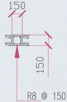
KERATAN X - X
