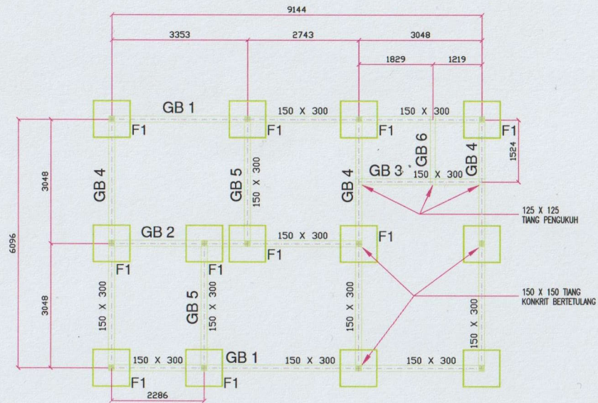
PELAN RASUK TINGKAT BAWAH DAN ASAS PAD
