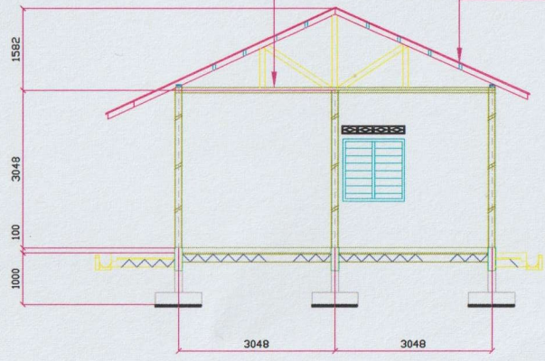
KERATAN Q - Q
