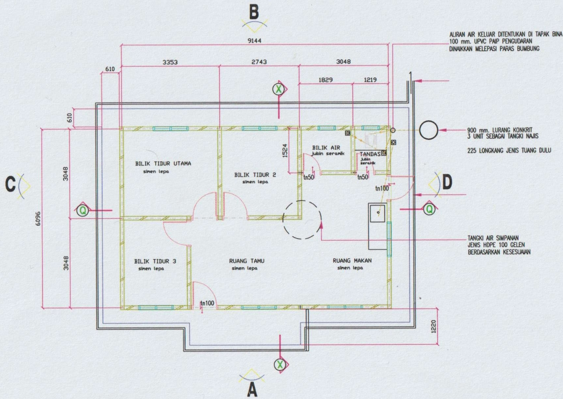
PELAN LANTAI
