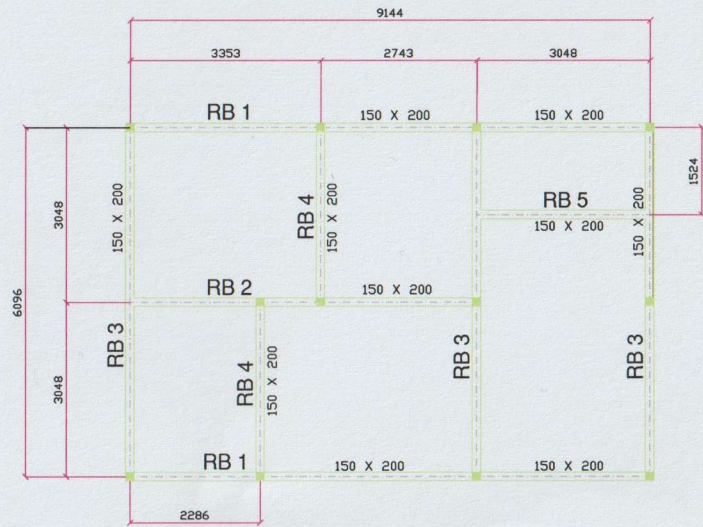
PELAN RASUK ALANG
